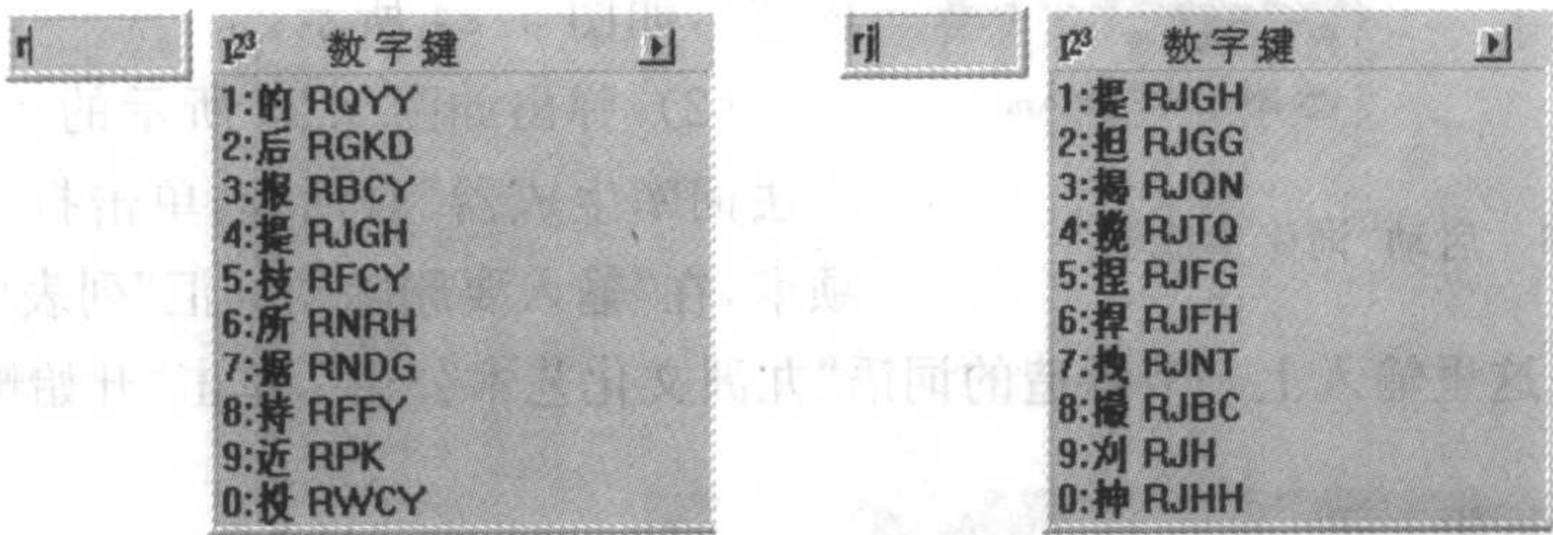
图 5.21 98 版的汉字编码提示功能
